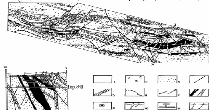
3-rasm. Marjonbuloq koni. Gorizont 816 geologik sxematik rejasi [2, 3]
