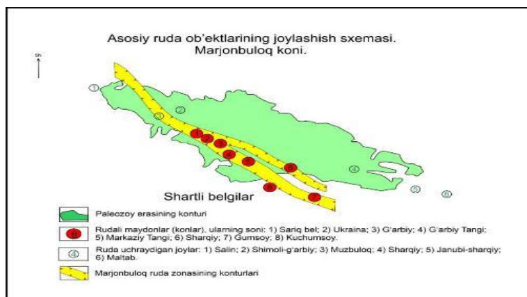
1-rasm. Marjonbuloq konidagi asosiy ruda ob'ektlarining sxematik xaritasi.
