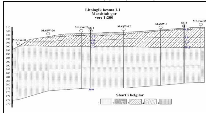
2-rasm. I-I chizig'i bo'yicha litologik kesim
