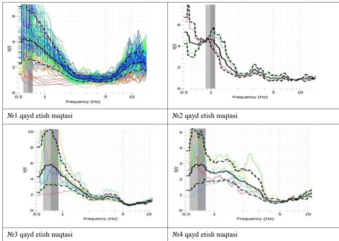
3-rasm. 1- 4 qayd etish nuqtalari uchun HVSr spektrlari.
