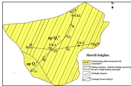
1-rasm. Termiz shahrining geologik-litologik xaritasi.
