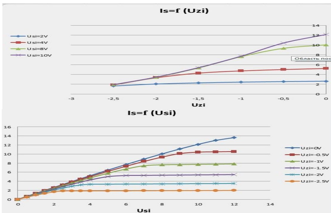
4-rasm. Xarakteristika tikligini hisoblashdan foydalanib tuzilgan grafik
