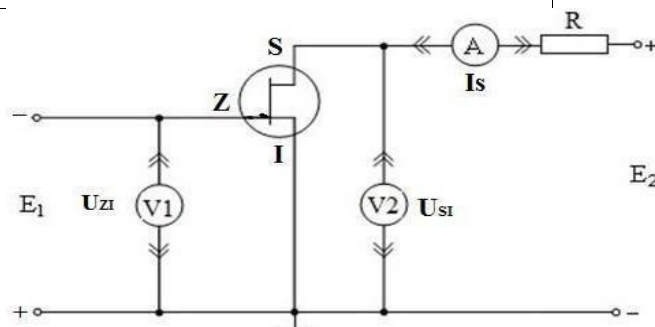
1-rasm. Umumiy istok ulanish sxemasidagi maydoniy tranzistorning uzatish va chiqish xarakteristikalar oilasini o'lash prinsipial sxemasi
